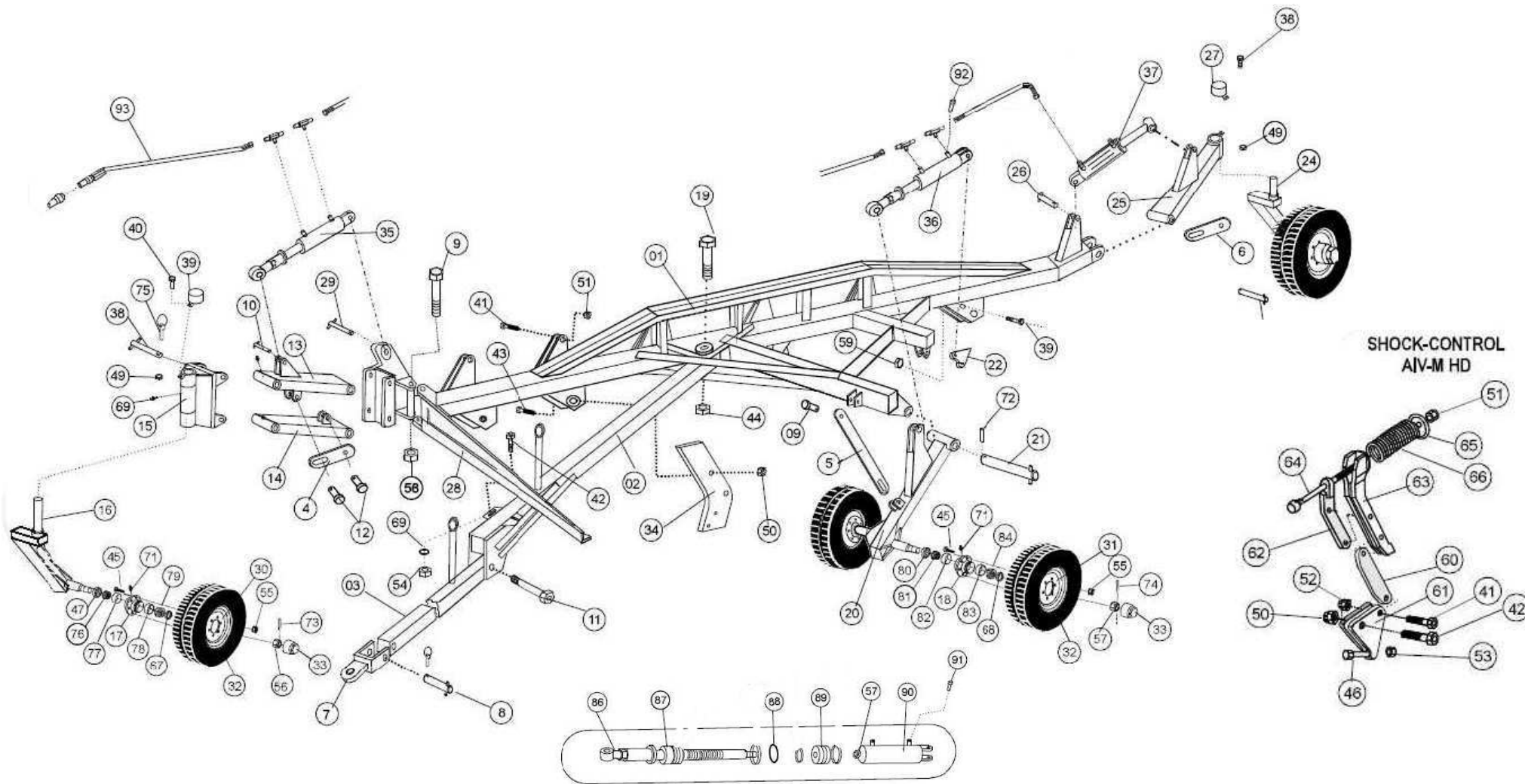
CILINDRO HIDRAULICO DIANTEIRO/INTERMEDIÁRIO E TRAZEIRO
